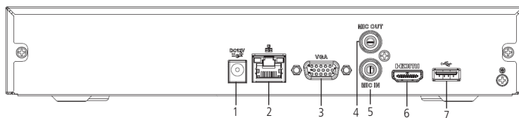
Painel posterior
